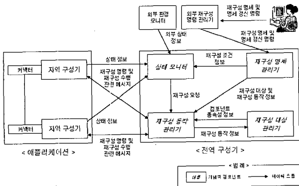
그림 9 재구성기의 개념적 모델
