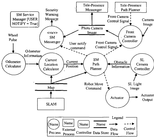
그림 5 SM을 위한 DFD 명세
