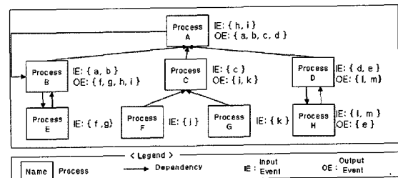
그림 11 프로세스 입/출력 의존 그래프 예제
