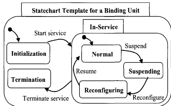
그림 4 휘처 바인딩 유닛의 행위 명세를 위한 스테이트차트 템플릿
