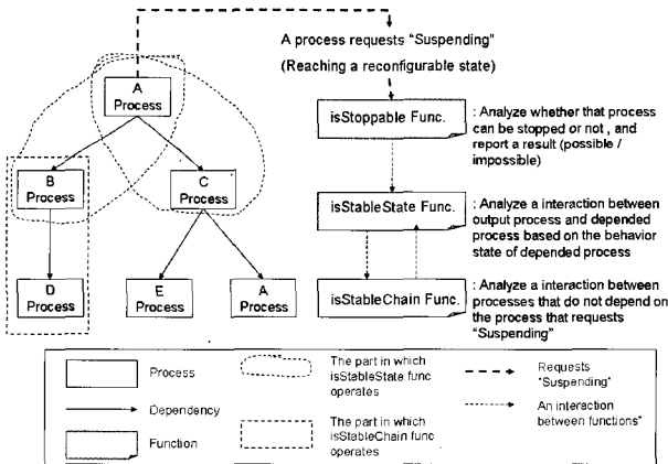
그림 12 프로세스 중지 가능성 판단 알고리즘 개요
