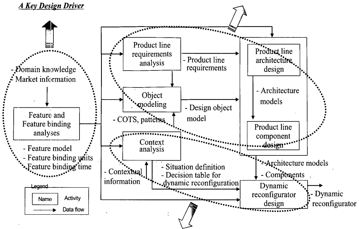
그림 1 접근 방법의 주요 활동
