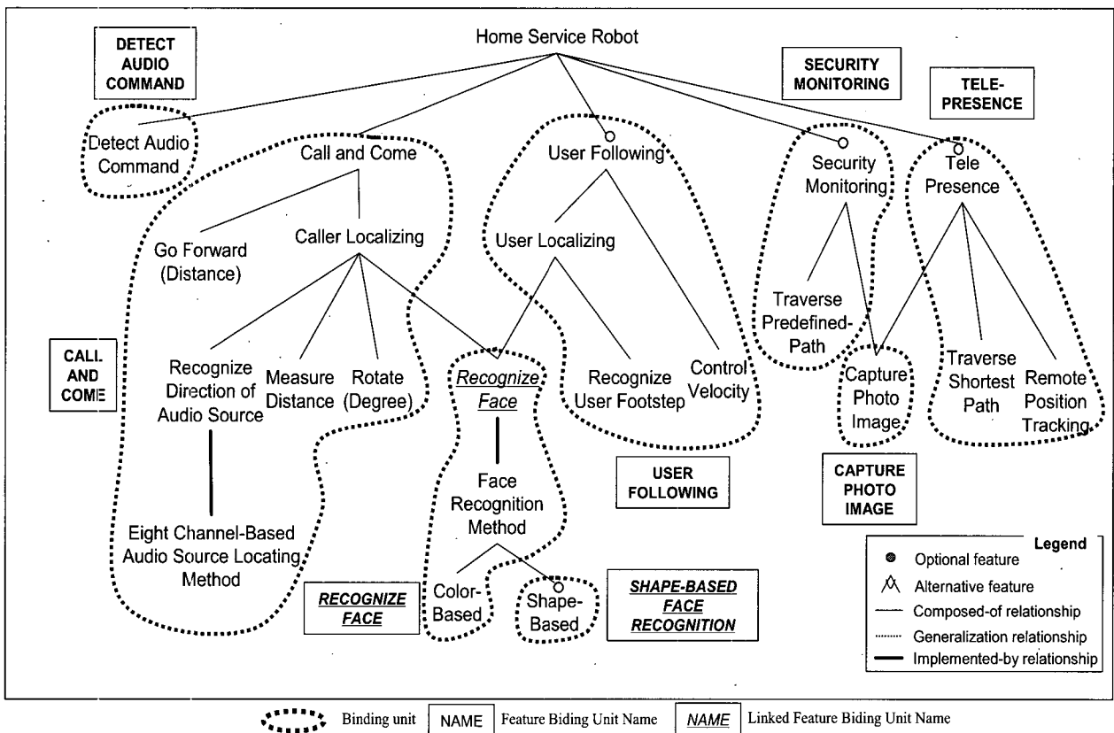
그림 2 HSR 프로젝트 라인의 휘쳐 모델과 바인딩 유닛 식별
