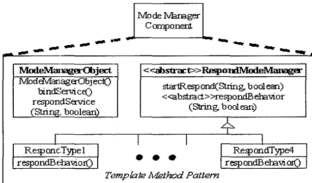
그림 7 Mode Manager의 컴포넌트 명세
