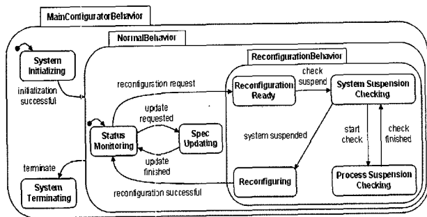
그림 10 전역 구성기 행위 명세
