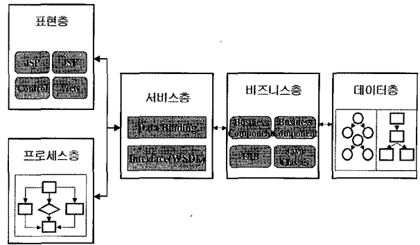
그림 3 서비스 중심 애플리케이션을 이루는 계층
