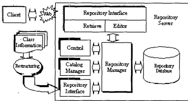
그림 2 저장소 구조
