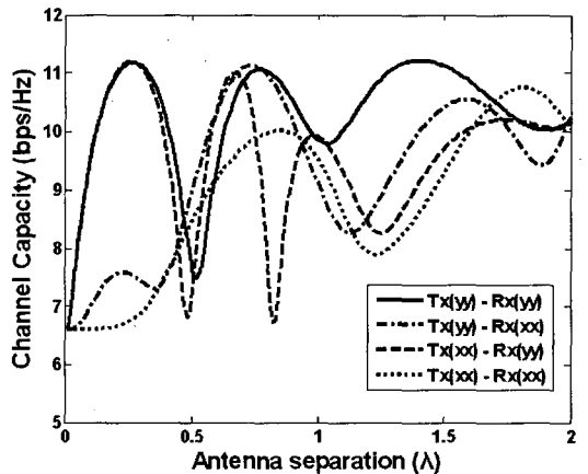
그림 8. LOS 위치에서 송수신기 방향 조합에 따른 채널 용량 비교 Fig. 8. Comparison of channel capacities for four different direction combinations at LOS.
