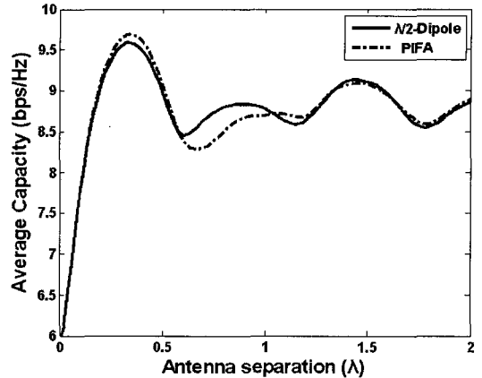
그림 10. MIMO 시스템의 안테나 이격 거리에 대한 평균 채널 용량
