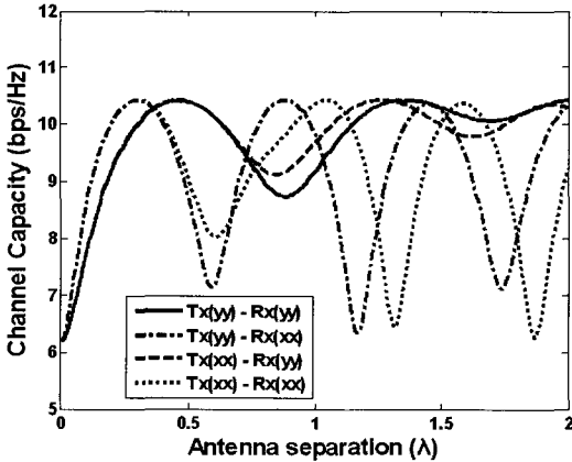
그림 9. NLOS1 위치에서 송수신기 방향 조합에 따른 채널 용량 비교
