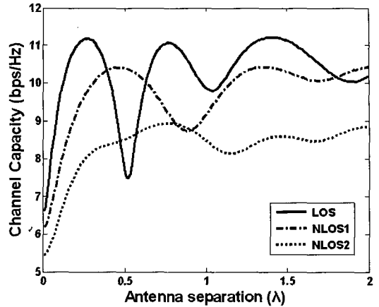
그림 7. 세 개의 수신기 위치에서 안테나 이격 거리에 따른 채널 용량 Fig. 7. Channel capacity with respect to antenna separation at three different receiver positions.
