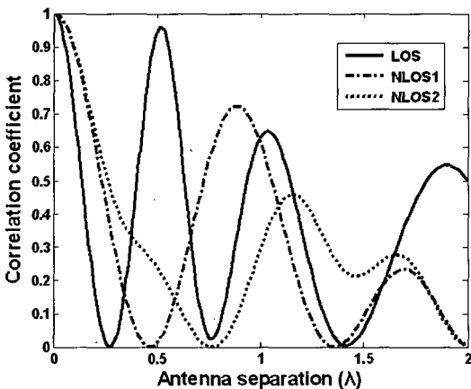
그림 6. 세 개의 수신기 위치에서 안테나 이격거리에 따른 상관 계수 Fig. 6. Correlation coefficient with respect to antenna separation at three different receiver positions.
