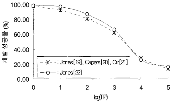
(그림 3) log(FP)와 개발 성공률 관계
