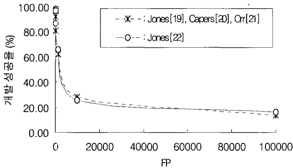
(그림 2) 소프트웨어 규모와 개발 성공률 관계
