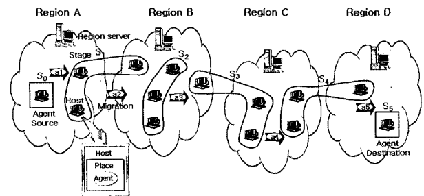
(그림 1) 단계군으로 구성된 이동 에이전트 컴퓨팅 환경
