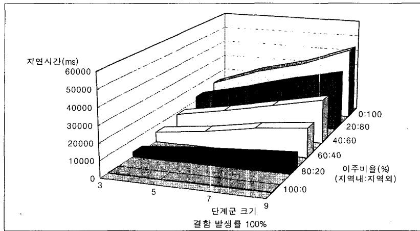
(e) 결함 발생률이 100% 인 경우
