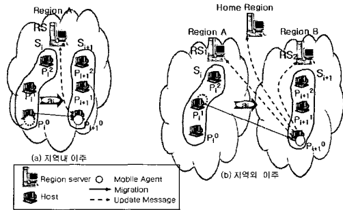
(그림 3) 이동 에이전트 이주 과정
