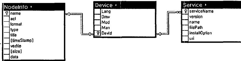
(그림 7) 매니저 데이터베이스 스키마
