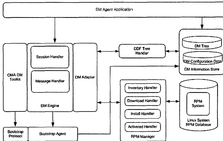
(그림 8) ThinkSync DM-SoftMan 에이전트 구현 구조
