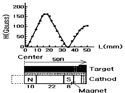
그림 6. 캐소드의 자계특성.
