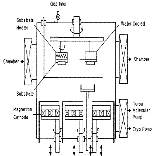
그림 1. Magnetron Sputtering 장치개략도.
