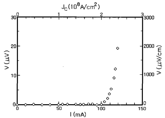
그림 2. 임계전류 특성.
