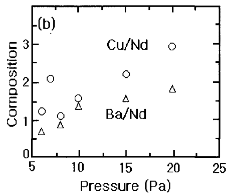
그림 4. 박막조성비의 스퍼터 가스압력의존성.
