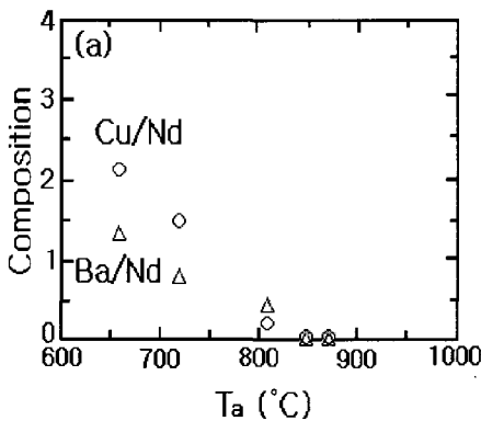
그림 3. 박막 조성비의 기판온도의존성.
