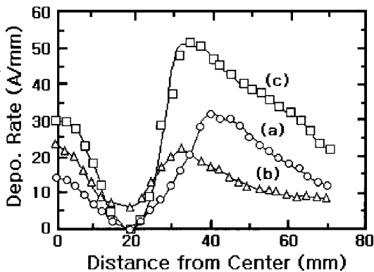
그림 5. 증착 Rate 변화.
