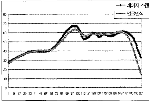
Fig. 8. 기기 보완 전 대상 2의 비침점 수직단면 오차비교
