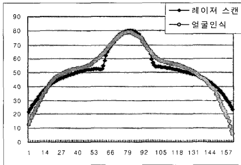
Fig. 12. 기기 보완 전 대상 2의 비침점 수평단면 오차비교
