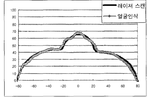
Fig. 13. 기기 보완 후 대상 2의 비침점 수평단면 오차비교
