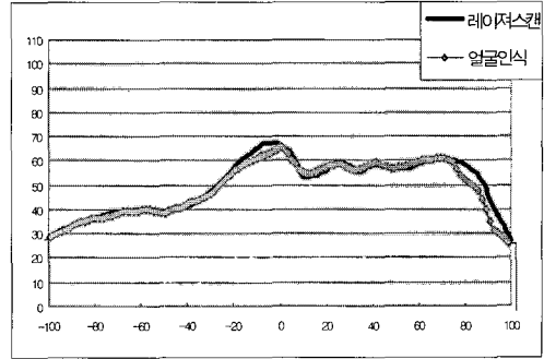
Fig. 9. 기기 보완 후 대상 2의 비침점 수직단면 오차비교
