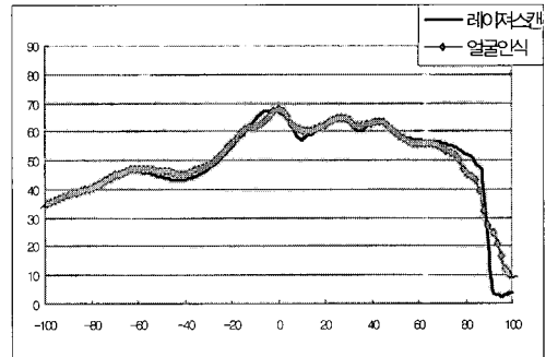
Fig. 7. 기기 보완 후 대상 1의 비침점 수직단면 오차비교
