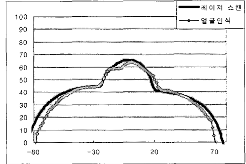
Fig. 11. 기기 보완 후 대상 1의 비침점 수평단면 오차비교
