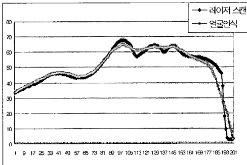
Fig. 6. 기기 보완 전 대상 1의 비침점 수직단면 오차비교
