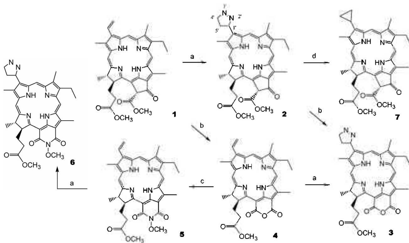
Scheme 1. a) \text{CH}_2\text{N}_2/\text{CH}_2\text{Cl}_2 ( 2 : 65%; 3 : 58%; 6 : 54%); b) \text{O}_2/\text{KOH}/\text{CH}_3\text{CH}_2\text{CH}_2\text{OH}/\text{Py}/\text{CH}_2\text{N}_2 ( 3 : 9%; 4 : 68%); c) \text{NH}_2\text{OH}\cdot\text{HCl}/\text{Py} ( 5 : 90%); d) o -DCB/ 180^\circ\text{C} ( 7 : 80%).
