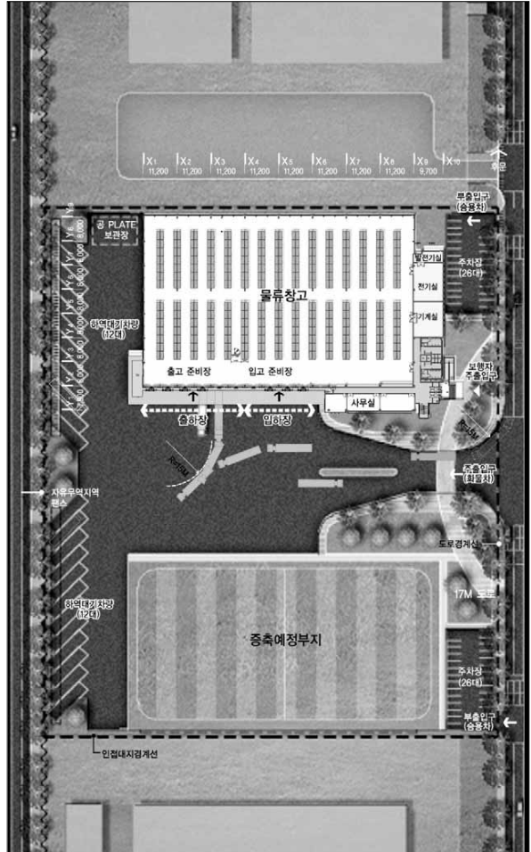
1층 평면도(물류창고)
