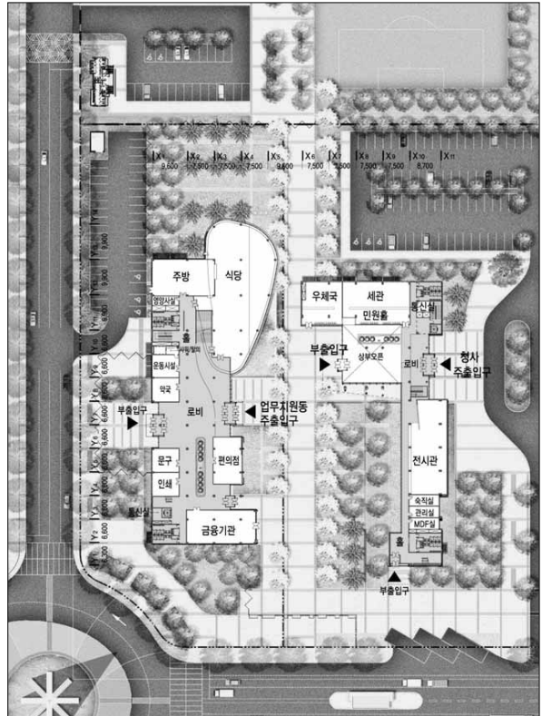
1층 평면도(업무청사동)
