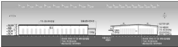
단면도(업무청사동)
