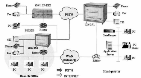
iDX-25/1 IP-PBX의 시스템 구성
