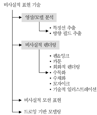
(그림 8) 비사실적 표현 기술 분류
