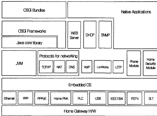
(그림 3) 홈 게이트웨이의 소프트웨어 구조
