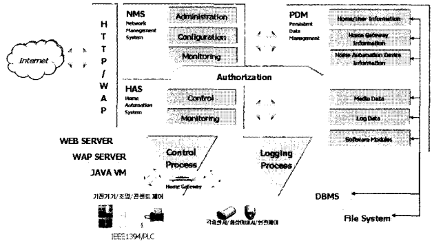
(그림 5) 관리 서버의 시스템 구조
