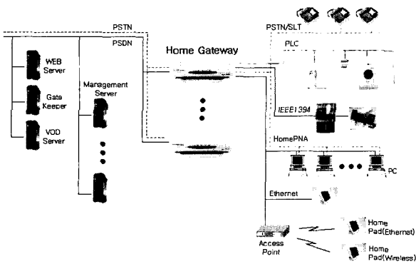
(그림 1) 홈 게이트웨이 시스템의 개요
