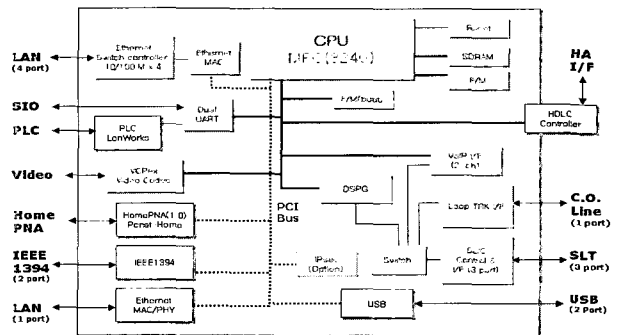
(그림 2) 홈 게이트웨이의 하드웨어 구조
