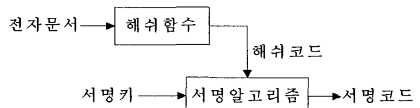
(그림 11) 식별정보서명시스템의 서명방식
