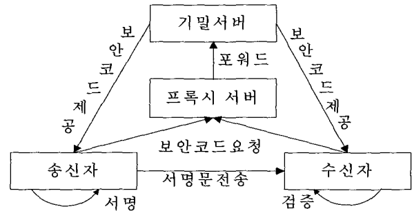
(그림 6) 식별정보서명시스템의 응용아키텍처
