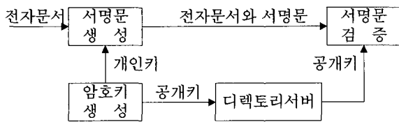
(그림 2) 디렉토리서버시스템의 서명 모델
