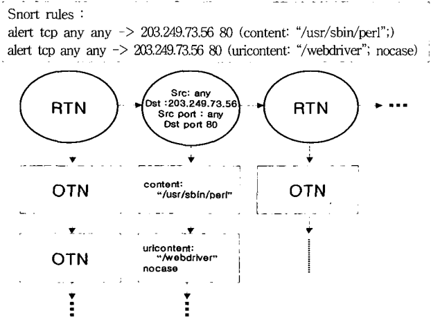
(그림 1) RTN and OTN 링크드 리스트 구조와 Snort 규칙
