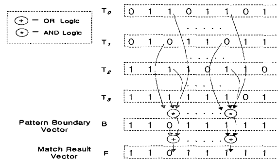
(그림 5) 매칭 발견 장치성능평가
