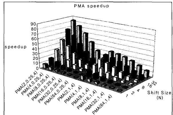
(그림 7) Shift size N , 메모리 접근 시간, Shift-OR 연산 시간 변화에 따른 PMA 속도증가율(배수)
