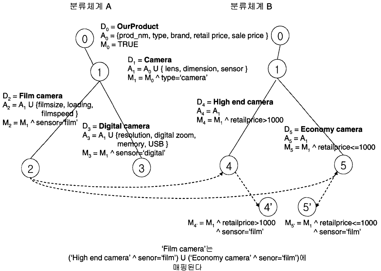
( 그림 8 ) 의미적 분류체계의 매핑
