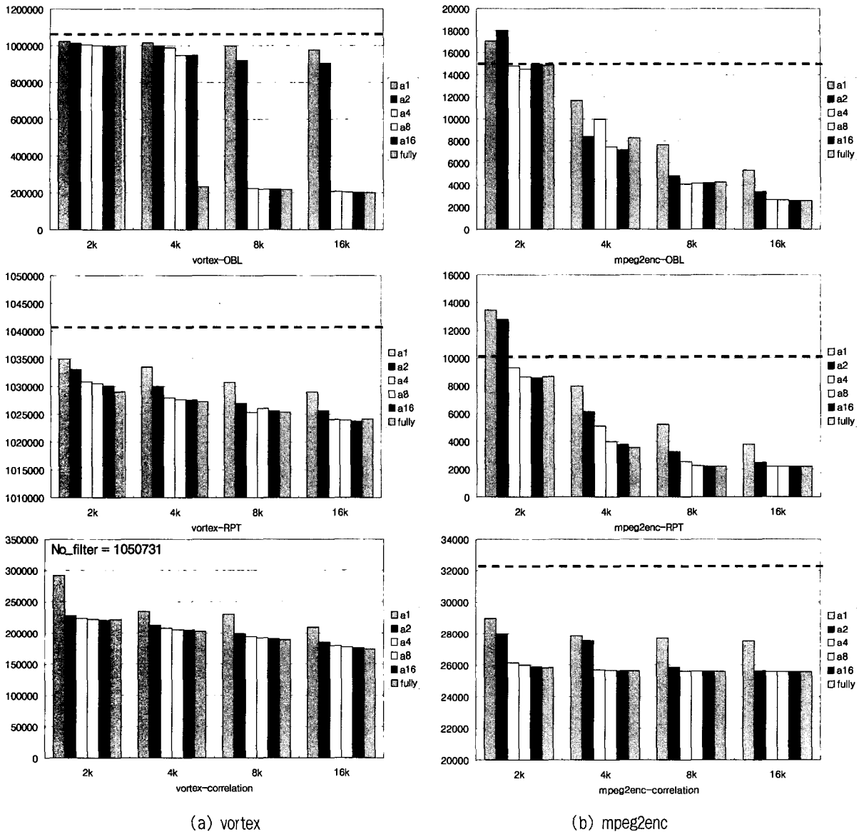
(그림 9) 선인출 전용 캐시의 크기별 캐시 미스 수 비교(메인 캐시 = 64K) (top : OBL, middle : RPT, bottom : correlation)
