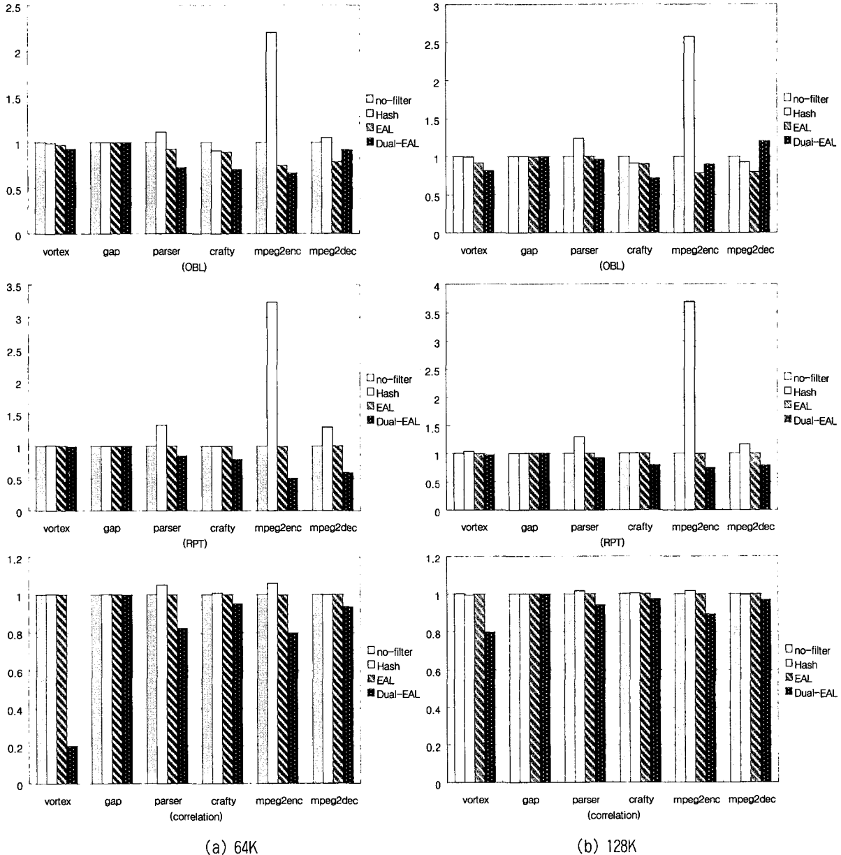
(그림 8) 벤치마크별 캐시 미스 수 (top : OBL, middle : RPT, bottom : correlation)
