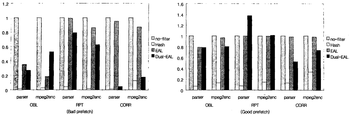
(그림 7) good과 bad 선인출 수 비교(좌측 : bad prefetch, 우측 : good prefetch)
