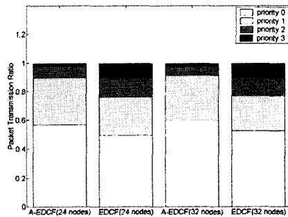
그림 8. 패킷 전송 비율로 나타난 적응형 EDCF와 EDCF의 우선순위 보장 비교(노드의 수가 24개, 32개인 경우)
