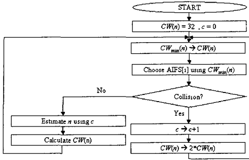
그림 3. 적응형 EDCF 동작의 순서도
