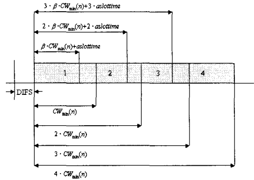
그림 5. 적응형 EDCAF의 AIFS의 결정
