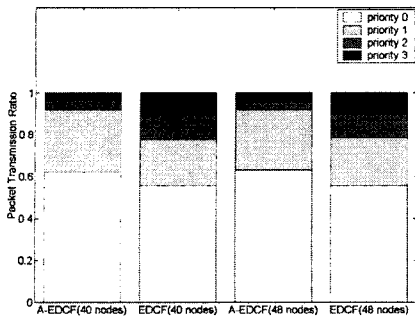
그림 9. 패킷 전송 비율로 나타낸 적응형 EDCF와 EDCF의 우선순위 보장 비교(노드의 수가 40개, 48개인 경우)
