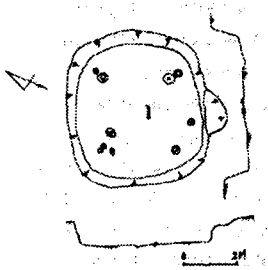
그림 17 암사동 제6호 움집터 평면도
