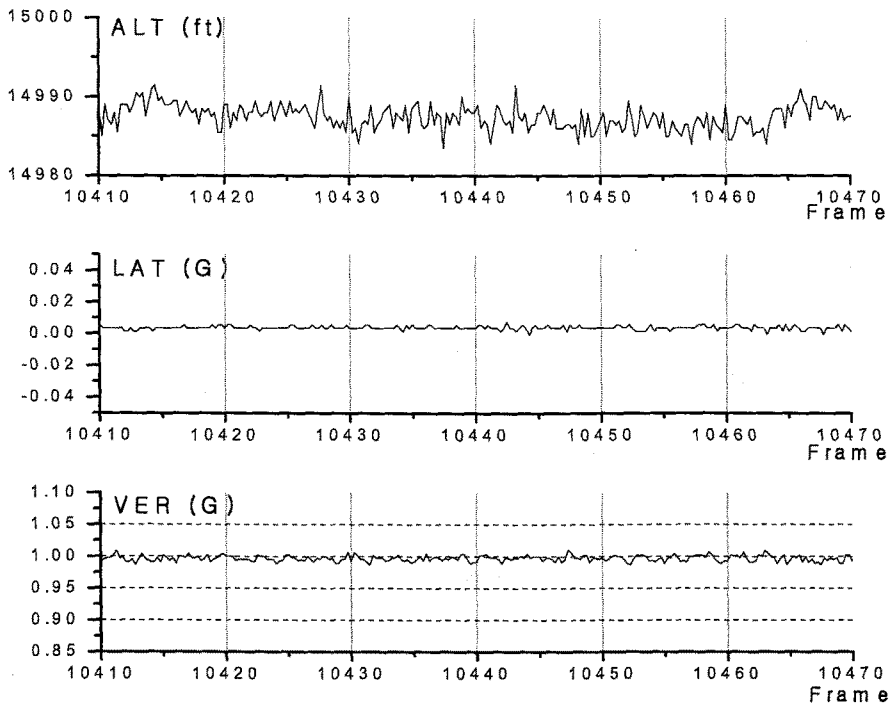
<그림 1> 수평순항비행 중 비행요란이 거의 없는 상태의 고도, 횡가속도, 수직가속도들의 변화
