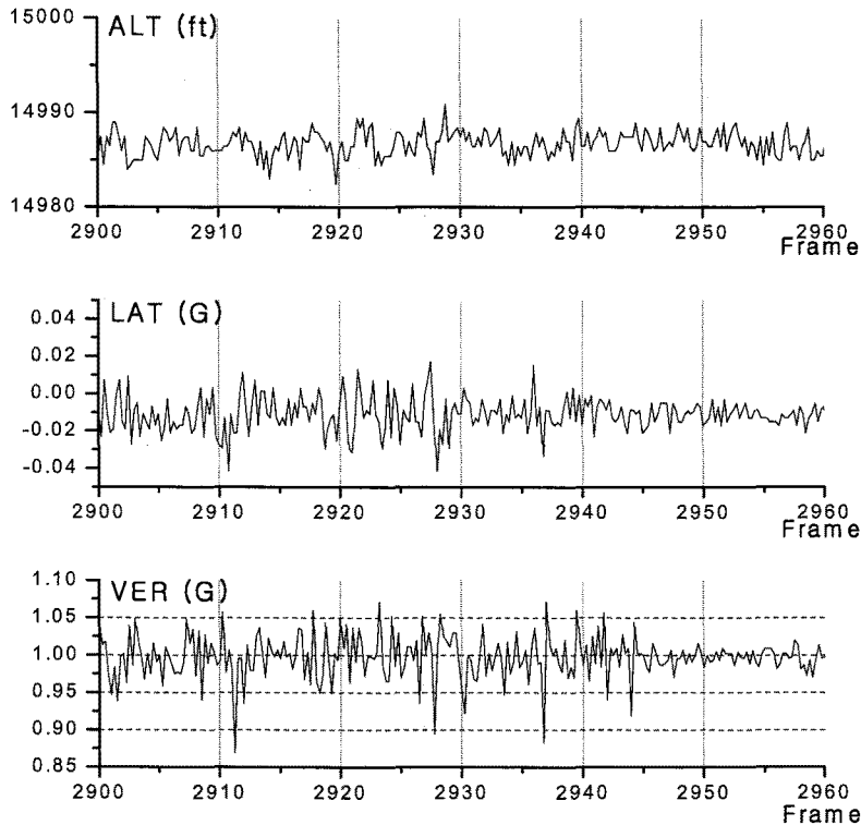
<그림 2> 수평순항비행 중 비행요란이 있었던 상태의 고도, 횡가속도, 수직가속도들의 변화
