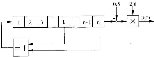
Fig. 4 PRBS generator
