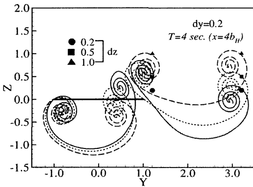
(a) OGE ( h=\infty )
