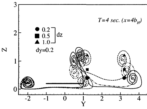
(b) IGE ( h=0.2 )
