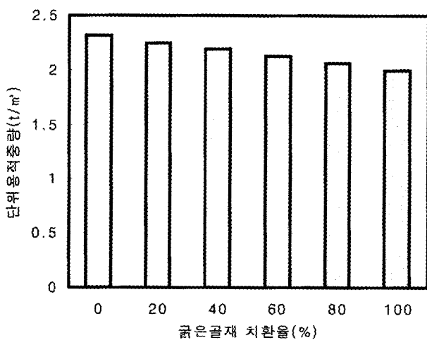
그림 4. 단위용적중량(잔골재 치환율 0%)
