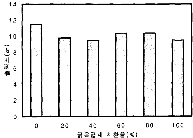
그림 2. 치환율에 따른 슬럼프(잔골재 치환율 100%)
