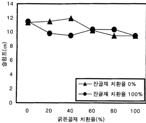
그림 3. 잔골재 치환율에 따른 슬럼프
