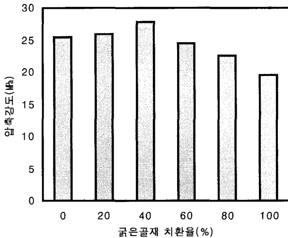
그림 8. 압축강도 (잔골재 치환율 100%)
