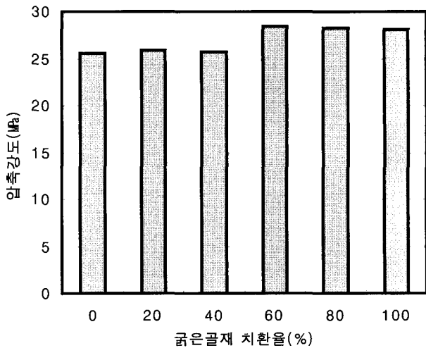
그림 7. 압축강도 (잔골재 치환율 0%)
