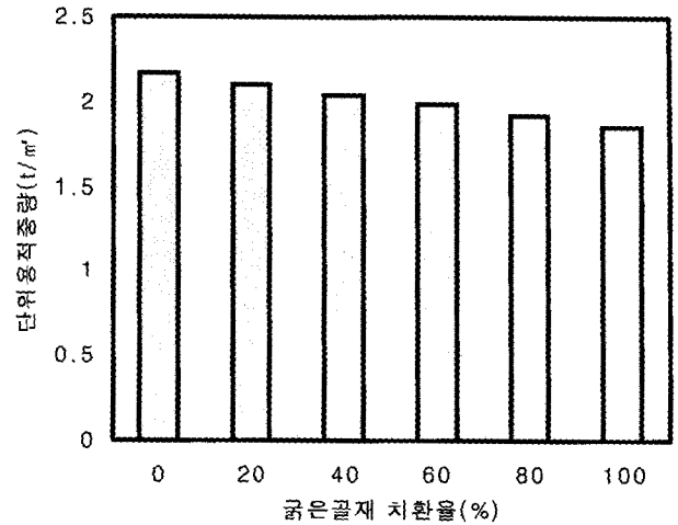
그림 5. 단위용적중량(잔골재 치환율 100%)
