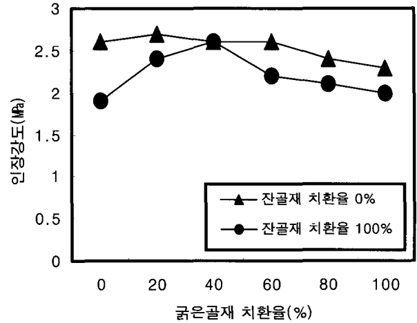
그림 12. 잔골재 치환율에 따른 인장강도
