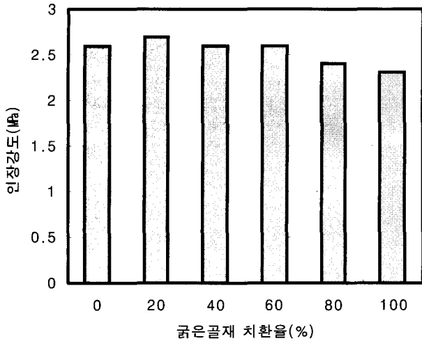
그림 10. 인장강도 (잔골재 치환율 0%)
