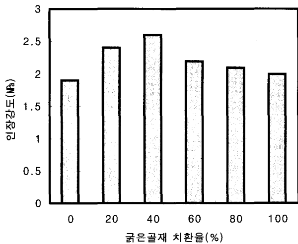
그림 11. 인장강도 (잔골재 치환율 100%)
