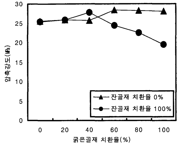
그림 9. 치환율에 따른 압축강도
