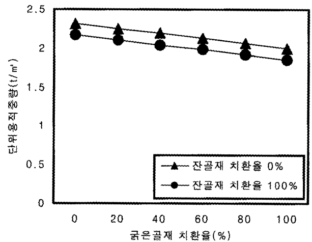
그림 6. 잔골재 치환율에 따른 단위용적중량
