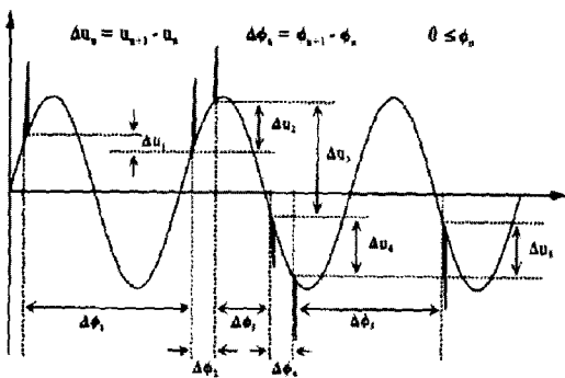
그림 1. PSA 분석기법의 개념. Fig. 1. Concept of PSA.
