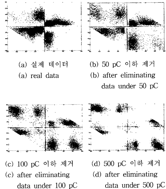
그림 4. 계면 전기트리에 대한 측정감도 차이 효과. Fig. 4. Effects of measuring sensitivity for the surface electrical tree.
