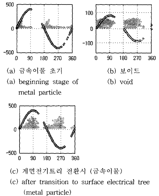
그림 2. 측정된 부분방전의 PRPD 패턴 예. Fig. 2. Examples of PRPD patterns for the measured partial discharges.
