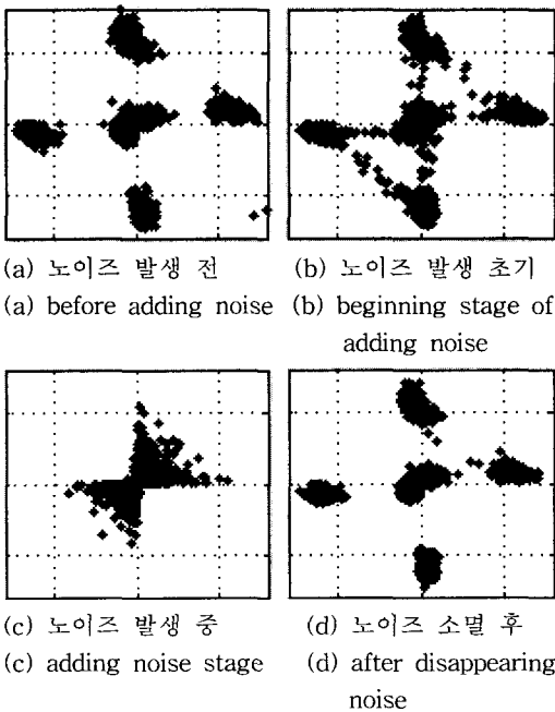
그림 7. 노이즈 발생 전후의 PSA 패턴 비교. Fig. 7. Comparison of PSA patterns with and without adding noise.
