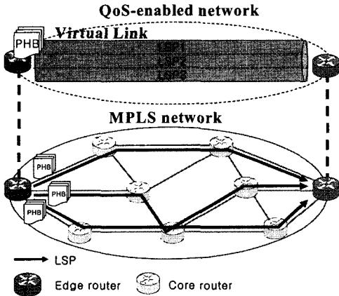
그림 3. 가상 링크로 구성된 논리적인 QoS 네트워크
