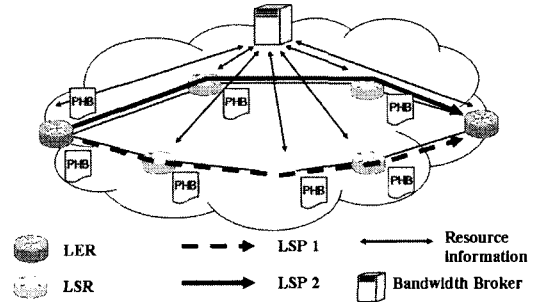
그림 1. 차등화 서비스를 통한 QoS 보장 방안 모델
