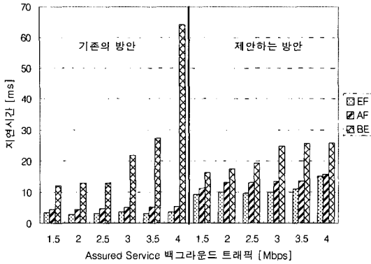
그림 7. AF 트래픽 변화에 따른 서비스별 지연시간
