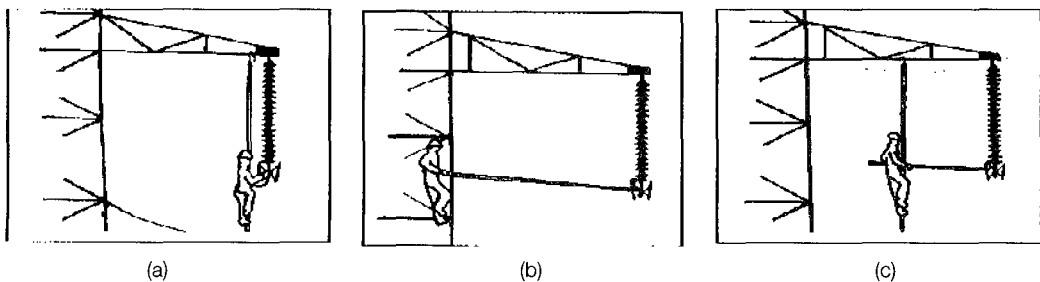
그림 1 활선 공법의 개념도
