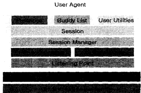
그림 7. 사용자 에이전트의 구조 Fig 7. Architecture of user agent
