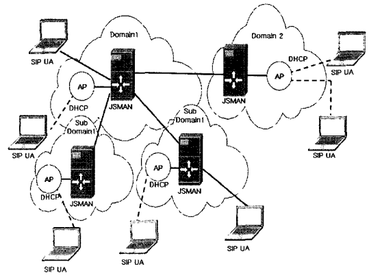
그림 2. 전체적인 시스템 구조 Fig 2. Overall System Architecture
