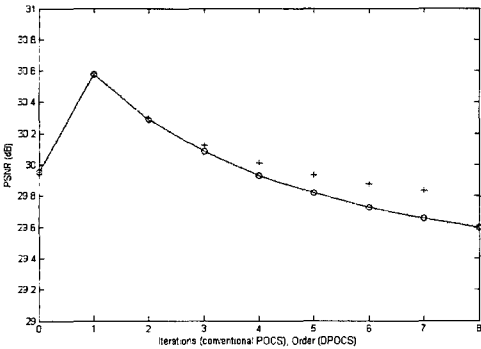
그림 6. 'Baboon' 영상에 대한 기존의 POCS 방식의 반복 회수와 제안된 DCT 영역에서의 POCS 방식의 차수에 대한 후처리된 영상의 PSNR 값 (기존의 POCS 방식: +점선, 제안된 DCT 영역에서의 POCS 방식: o 실선)
