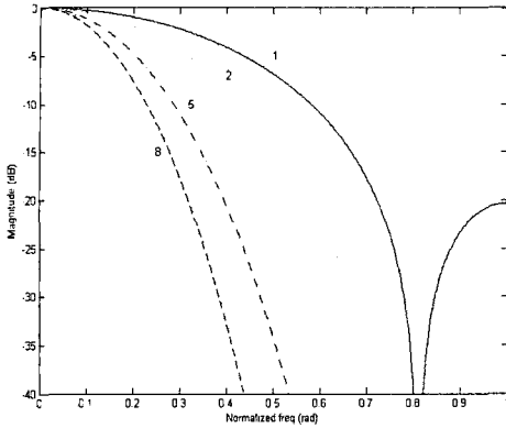
그림 2. \{v^{(k)}(m)\} 에 대한 주파수 응답 ( k=1,2,5,8 )
