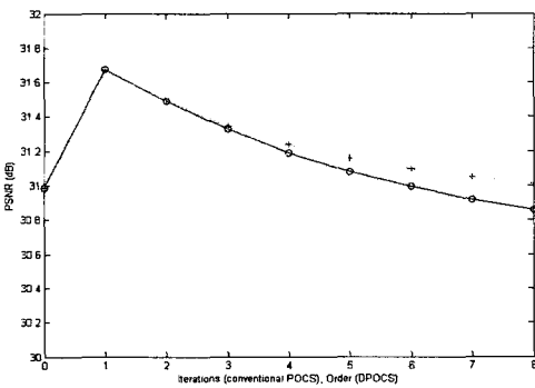
그림 7. 'Peppers' 영상에 대한 기존의 POCS 방식의 반복 회수와 제안된 DCT 영역에서의 POCS 방식의 차수에 대한 후처리된 영상의 PSNR 값 (기존의 POCS 방식: +점선, 제안된 DCT 영역에서의 POCS 방식: o 실선)
