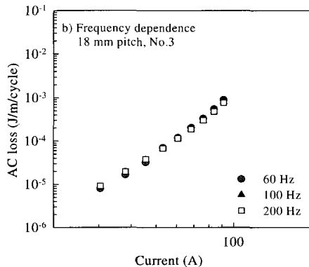
그림 4. Bifilar-코일에서 교류손실.
