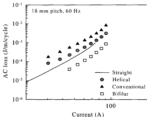
그림 5. 코일형 한류소자의 교류손실. Fig. 5. AC losses in the fault current limiting elements of a coil type.
