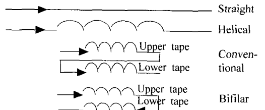
(a) 코일형 한류소자의 결선
