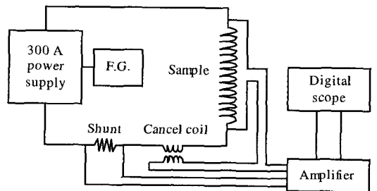
그림 2. 실험장치.
