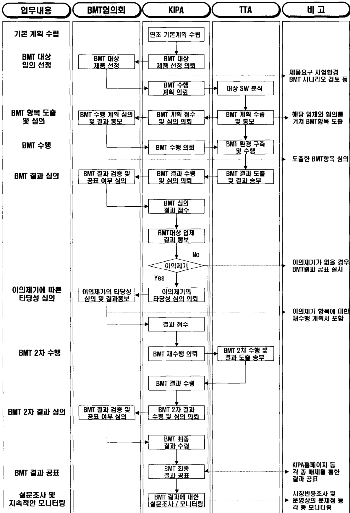
그림 1 S/W 벤치마크테스트 결과 공표 프로세스
