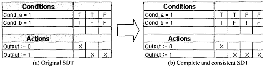
그림 5 f_X_Valid 를 위한 SDT의 완전성과 일관성에 관한 예
