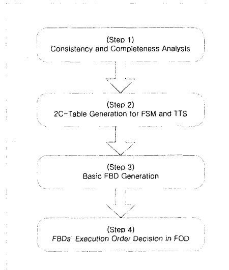
그림 4 FBD 생성의 전체 단계
