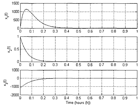
그림 2. 샘플링 시간 T=0.001(h) 에 대해서 아날로그 제어기 (실선)와 N=2을 가지는 디지털 제어기 (점선)를 사용한 폐루프 시스템의 시간 응답.
