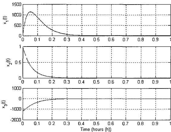
그림 1. 샘플링 시간 T=0.001(h) 에 대해서 아날로그 제어기 (실선)와 N=1을 가지는 디지털 제어기 (점선)를 사용한 폐루프 시스템의 시간 응답.
