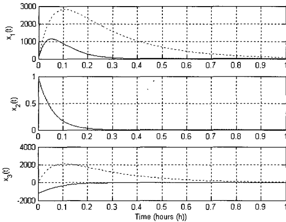
그림 3. 샘플링 시간 T=0.1(h) 에 대해서 아날로그 제어기 (실선)와 N=2 를 가지는 디지털 제어기 (점선)를 사용한 페루프 시스템의 시간 응답.
