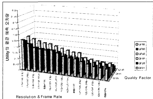
그림 9 콘텐츠 버전 별 유틸리티의 평균 예측 오차량
