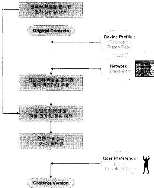
그림 7 동적 동영상 적응변환 시나리오
