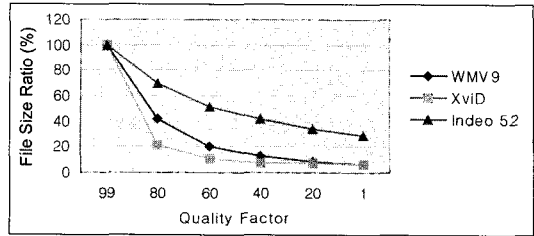
그림 2 코덱 별 Quality Factor에 따른 스트림 크기의 변화율
