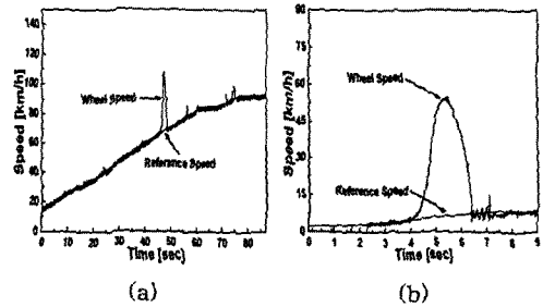
그림 5. 슬립과 슬라이드 발생. Fig. 5. Slip and slide occurrence.
