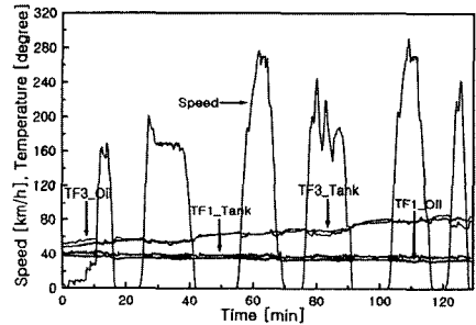
그림 11. 주변압기 과온 검지. Fig. 11. Over-temperature detection of main transformer.
