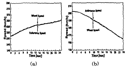
그림 6. 프로그램 수정후의 슬립과 슬라이드. Fig. 6. Slip and slide after program adjustment.
