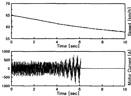
그림 9. 전동기 전류에 의한 고장진단. Fig. 9. Fault diagnosis using motor current.
