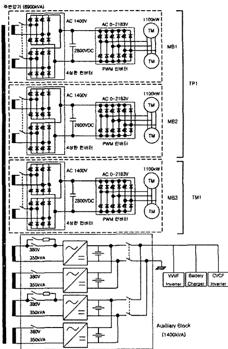
그림 1. 주회로 시스템. Fig. 1. Main circuit system.
