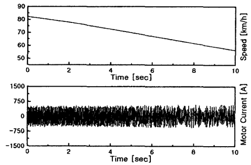
그림 10. 정상시의 전동기 전류. Fig. 10. Motor Current in case of ordinary condition.
