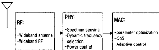
그림 4. Cognitive Radio의 블록도
