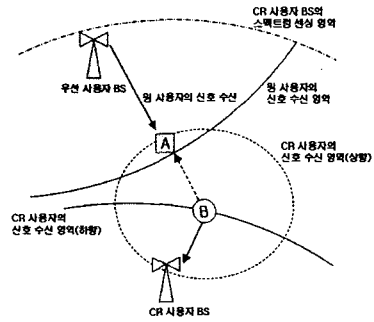
(b) CR BS에서의 스펙트럼 센싱 영역 확장
