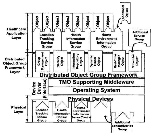
(그림 4) 분산객체그룹 프레임워크 기반의 헬스케어 홈 서비스 시스템 구조
