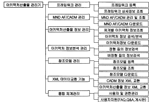
(그림 1) 아키텍처산출물 관리시스템 기능 구성도
