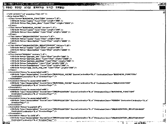
(그림 2) CADM의 메타모델 XML 교환
