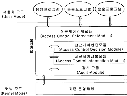
(그림 11) Secusys 보안커널 구조
