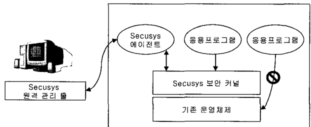
(그림 9) Secusys 시스템 구조
