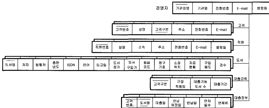
(그림 12) 재산 객체 속성구조 다이어그램
