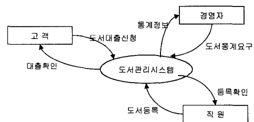
(그림 9) 컨텍스트 다이어그램
