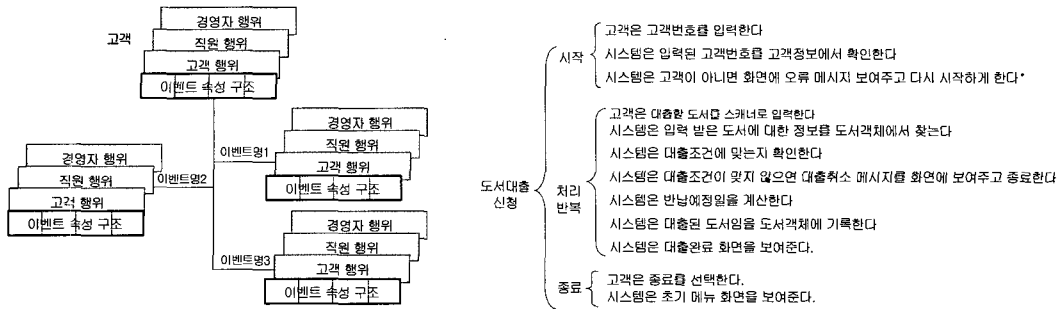
(a) 행위구조 다이어그램 (b) 행위 명세서
