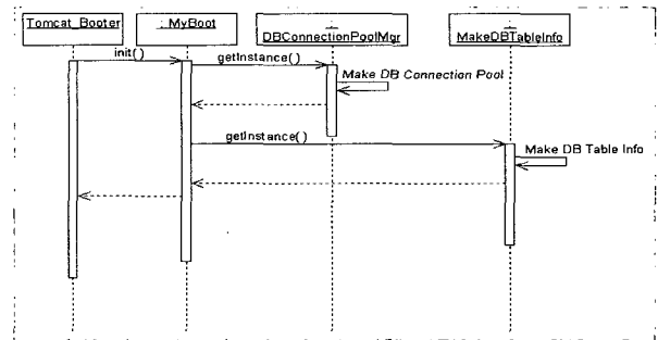
(그림 8) 부팅의 순서
