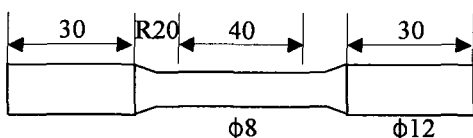
Fig. 1 Tensile test specimen
