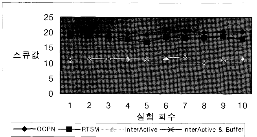
(그림 14) 세 가지 모델의 스킨값 비교
