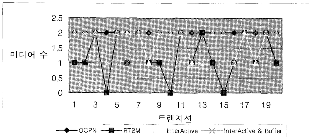
(그림 13) 세 가지 모델의 트랜지션 수행별 미디어 수
