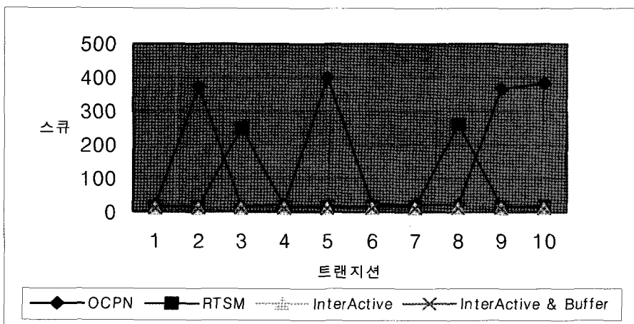
(그림 15) 트랜지션내의 세 가지 모델이 가지는 스킨값 비교
