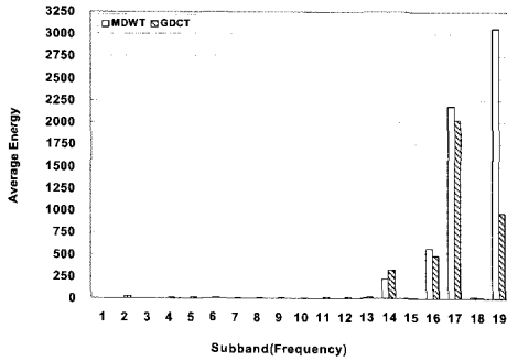
그림 9. DWT 영역에서 fringe의 에너지 분포 (최저주파 대역 제외) Fig. 9. energy distribution of fringe in DWT domain (with the exception of the lowest frequency subband)
