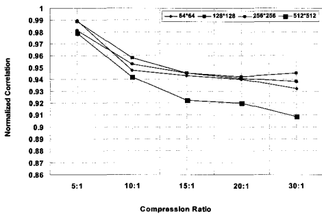
그림 14. MRME기반 부호화를 이용한 복원결과의 NC Fig. 14. NC of reconstructed result using encoding based MRME
