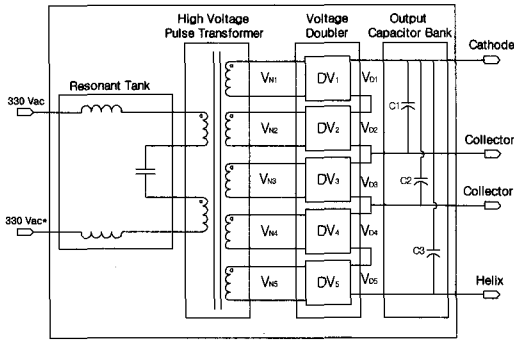
그림 2. 고압전원발생기 설계도
