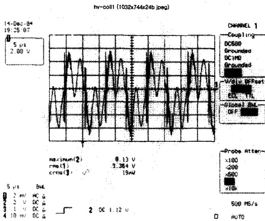
그림 5. Collector1 ripple
