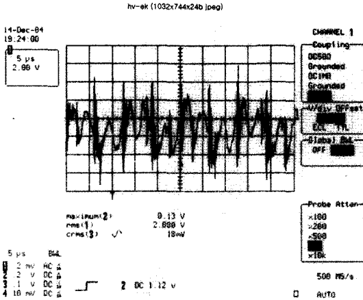
그림 4. Cathode ripple
