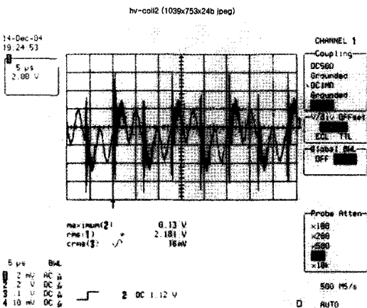
그림 6. Collector2 ripple
