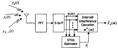
그림 2. 제안된 셀 간 간섭 제거 기법의 블록도
