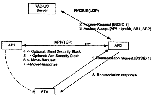
그림 4. 재연결(Reassociation) 시의 IAPP 메시지 교환
