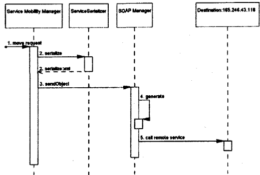
그림 4. 서비스 이동 전의 시퀀스 다이어그램 Fig 4. the sequence diagram before moving service
