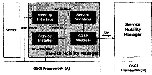
그림 2. OSGi 상의 서비스 이동 관리 시스템 Fig 2. Service mobility management system on OSGi
