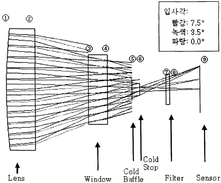
그림 4. PSICS 광학계 설계사양.
