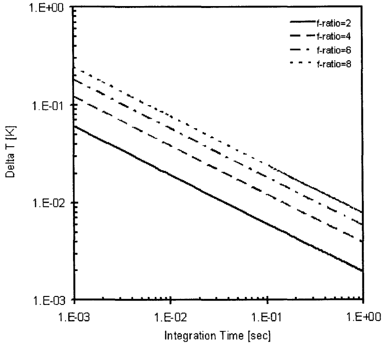
그림 3. 노출 시간에 따른 감도의 변화. 신호대 잡음비를 5로 관측할 수 있는 한계를 온도의 변화 값으로 표시하였다. 광학계의 f-비가 2 (실선으로 표시), 4 (긴 점선), 6 (길고 짧은 점선), 8 (짧은 점선)인 경우에 대해 각각 계산하였다.
