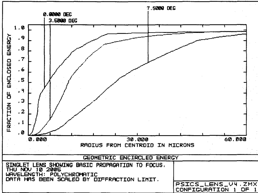
그림 6. 광학계 광점 이미지의 에너지 분포.
