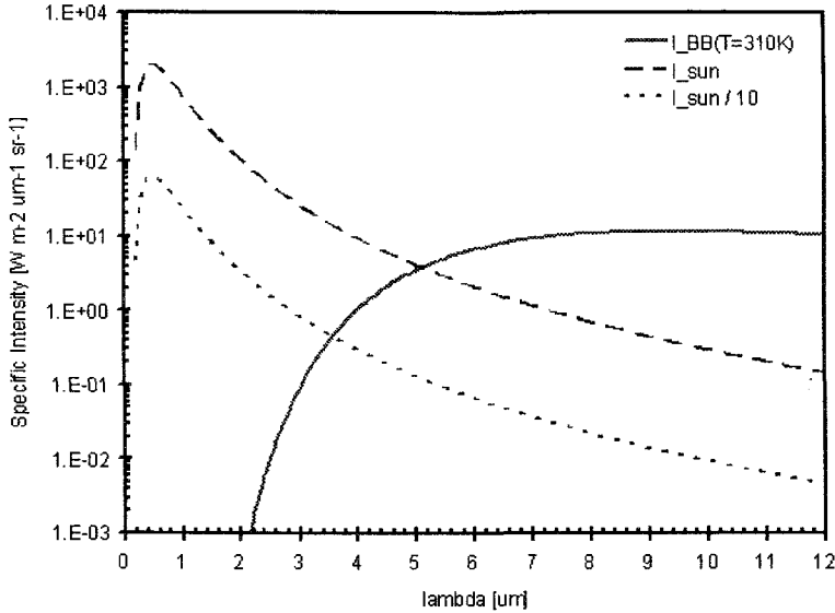
그림 2. 파장에 따른 태양의 복사 세기와 흑체 복사 세기의 비교. 실선은 표면 온도 310K인 흑체의 복사 세기를 보여주고, 긴 점선은 지구 표면에 있는 물체가 받는 태양의 복사 세기를 보여준다. 짧은 점선은 태양 복사 세기의 10%에 해당하는 값이다.
