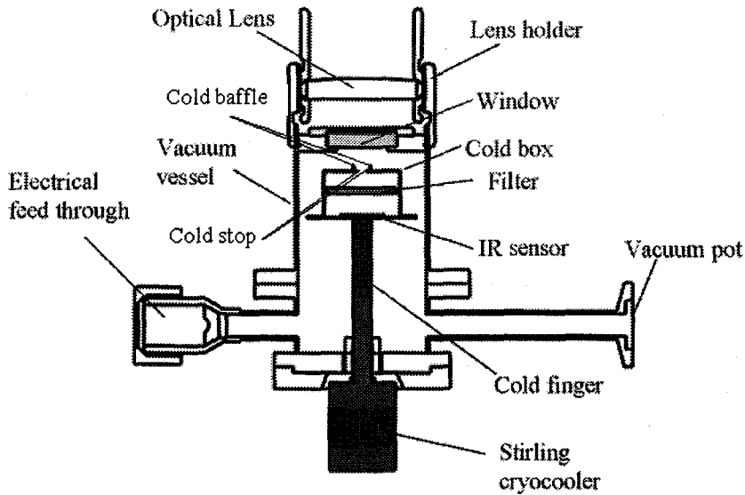
그림 1. PSICS의 개념 설계도(양형석 외 2005).
