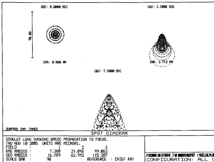
그림 5. PSICS 광학계의 광점 이미지 분포.
