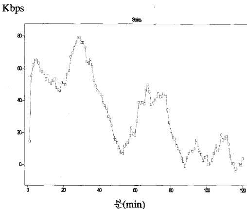
그림 6. 제안된 LMS-위너모델에 의한 자원의 예측 오차량
