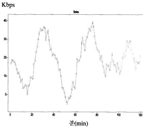
그림 5. 기존 위너모델에 의한 자원의 예측 오차량
