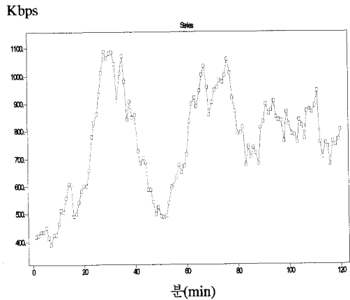
그림 2. 기존의 위너 모델에 의한 예측된 자원의 양
