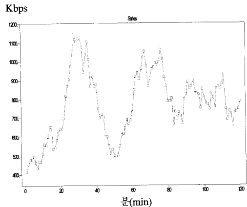
그림 3. 제안된 LMS- 위너모델에 의한 예측된 자원의 양
