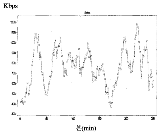
그림 9. 기존 위너모델에 의한 자원의 예측량
