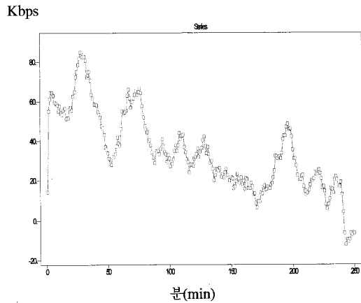
그림 13. LMS-위너모델에 의한 자원의 예측 오차량
