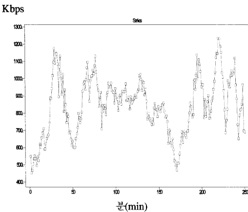
그림 11. ARMA 예측 모델에 의한 자원의 예측량
